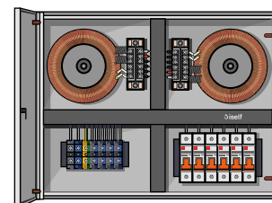
СИСТЕМА ПОДОГРЕВА ФУНКЦИОНАЛЬНЫХ ПАНЕЛЕЙ
